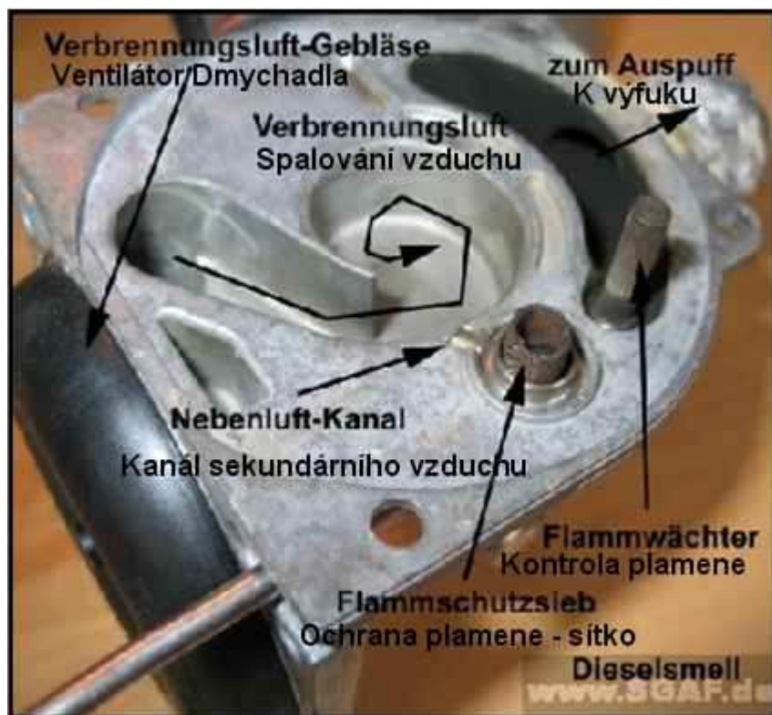
Obrázek 13: Výfuková část Dmychadla (vedení spalovacího vzduchu)
