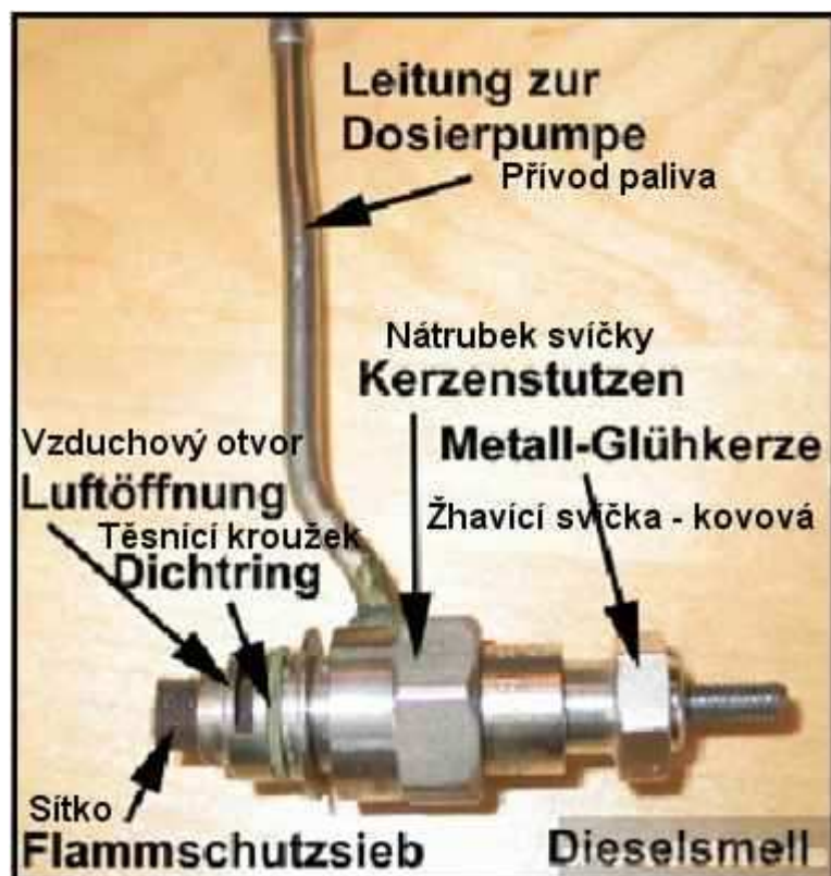
Obrázek 14: Sítko s žhavicí svíčkou a přívodem paliva
