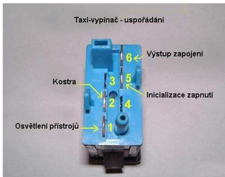
Obrázek 49: Uspořádání vypínače (zadní strana)
